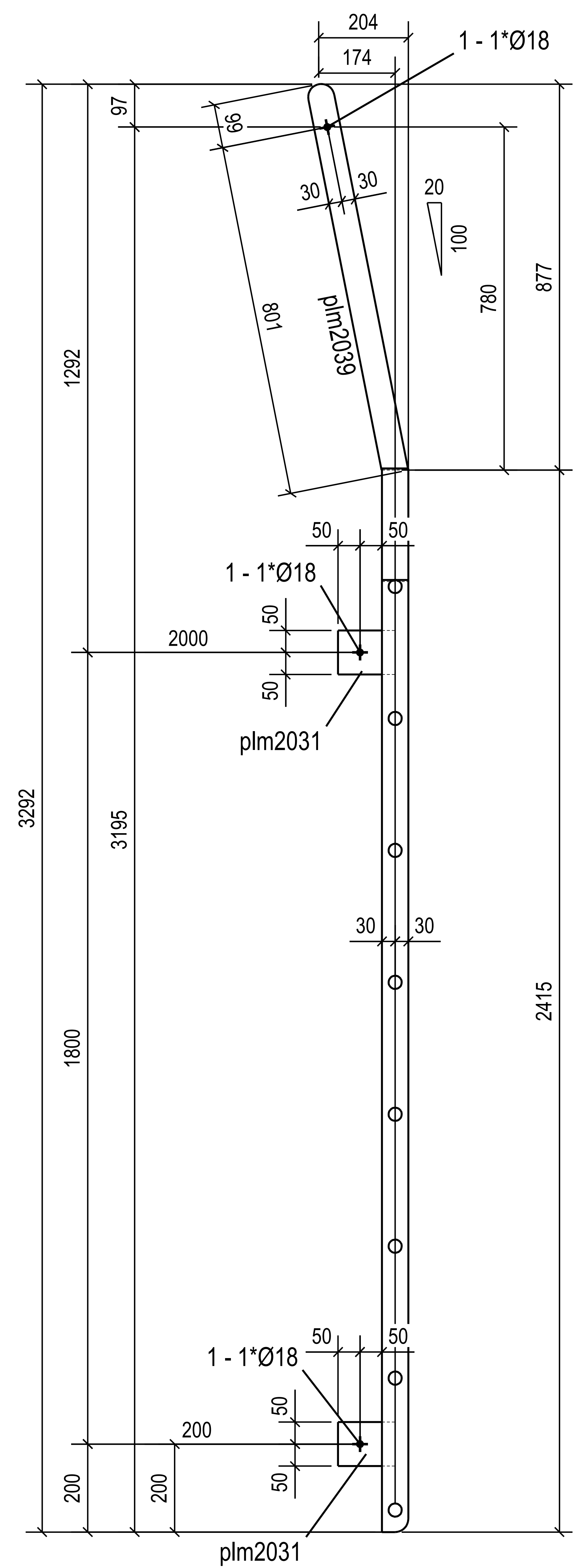
A SECTION A SCALE: 1:15
